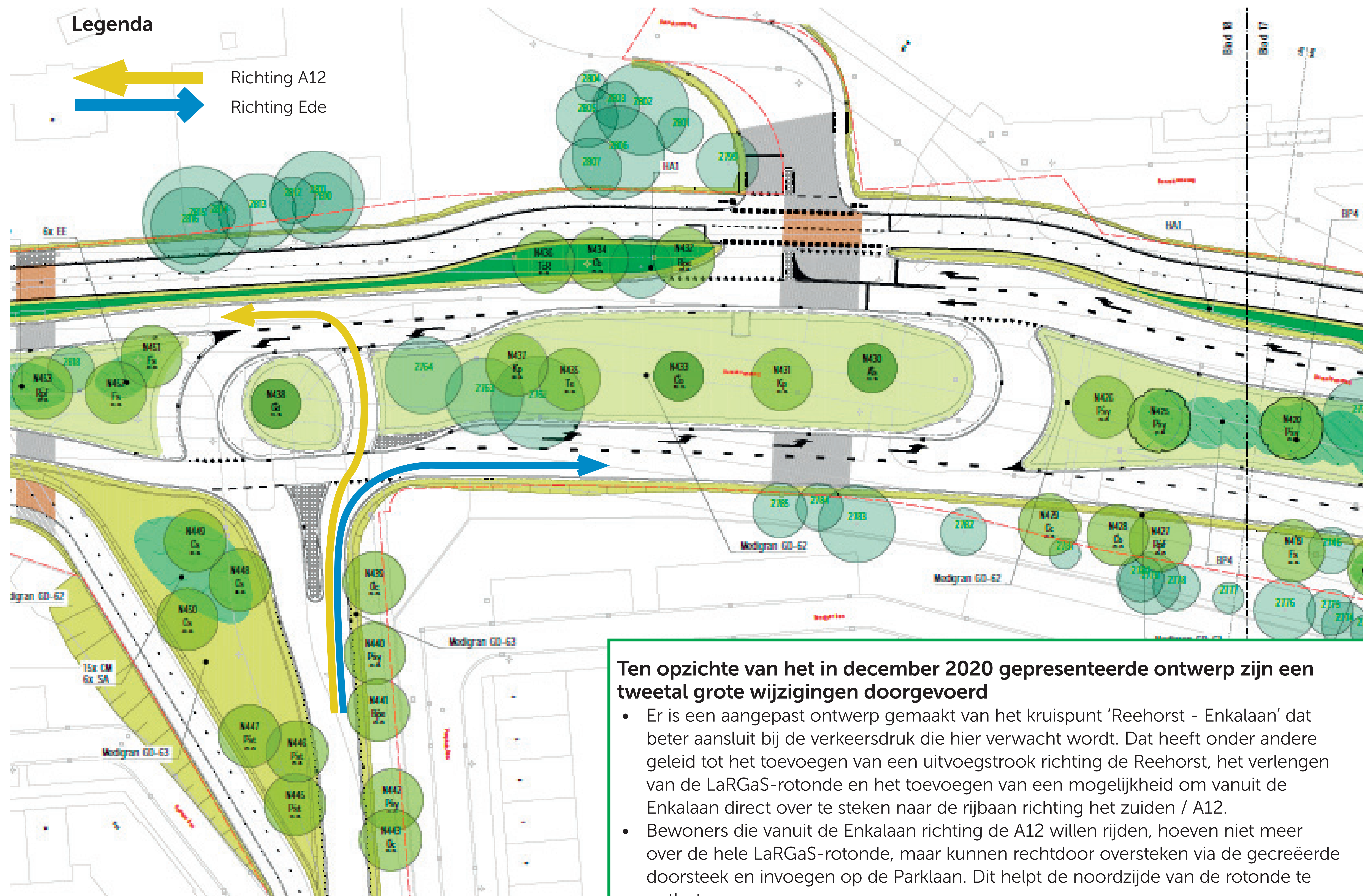
Het aangepaste ontwerp van kruispunt 'Reehorst - Enkalaan'
